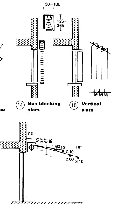
⑲ Adjustable awning
